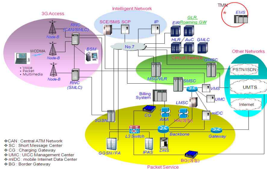
(그림 II - 6) 이동통신 망 구성도
