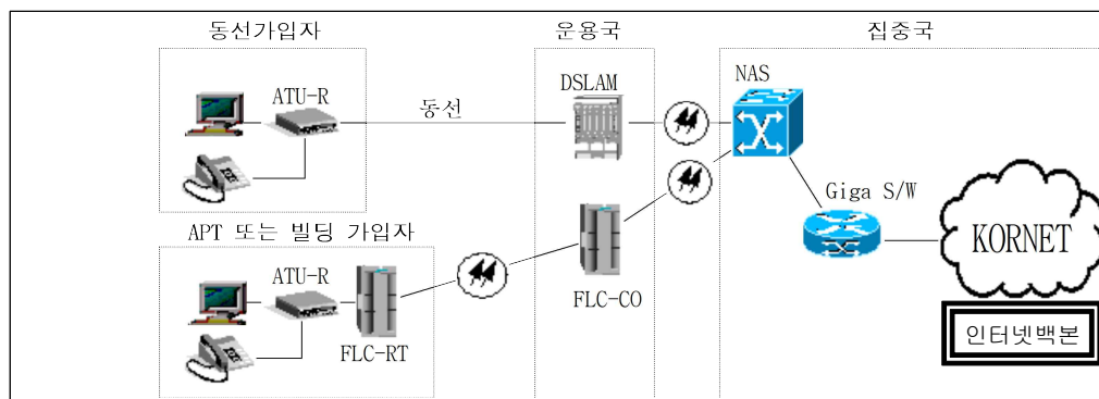
[그림 II - 2] 인터넷가입자접속망 구성도
