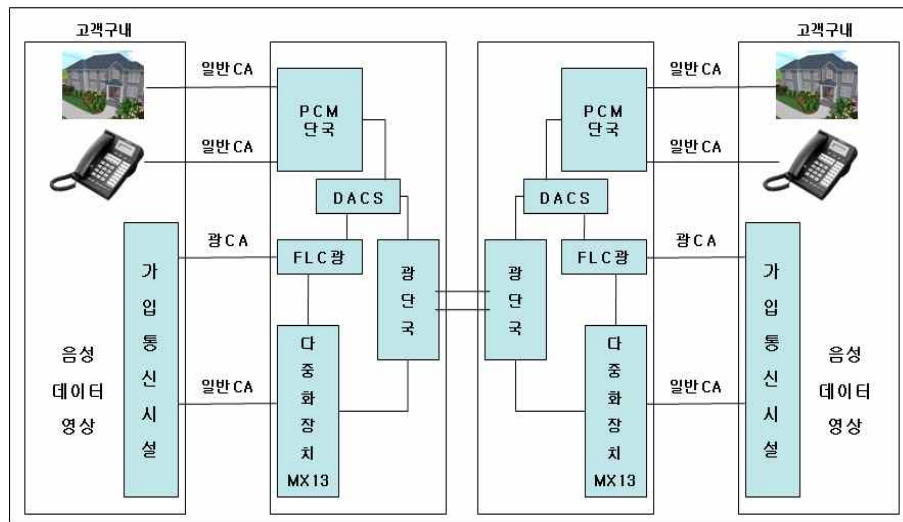
(그림 II - 5) 회선설비임대역무 망 구성도
