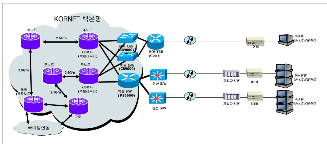
〔그림 II - 3〕 인터넷전용회선 망
