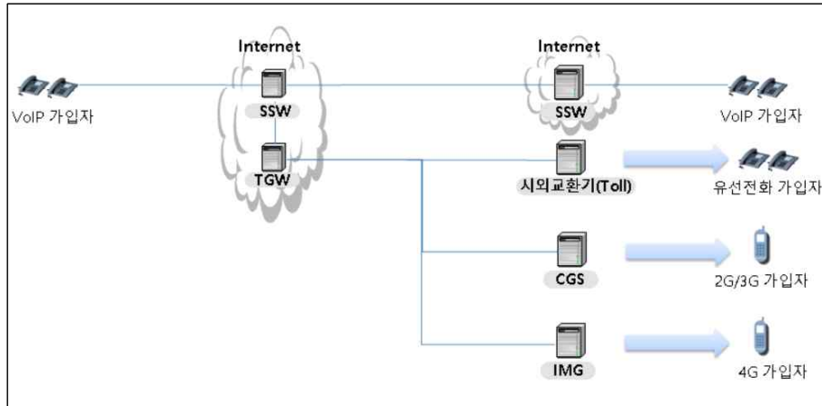
(그림 II-4) 인터넷전화 망 구성도
